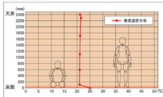
床暖房の垂直温度分布
